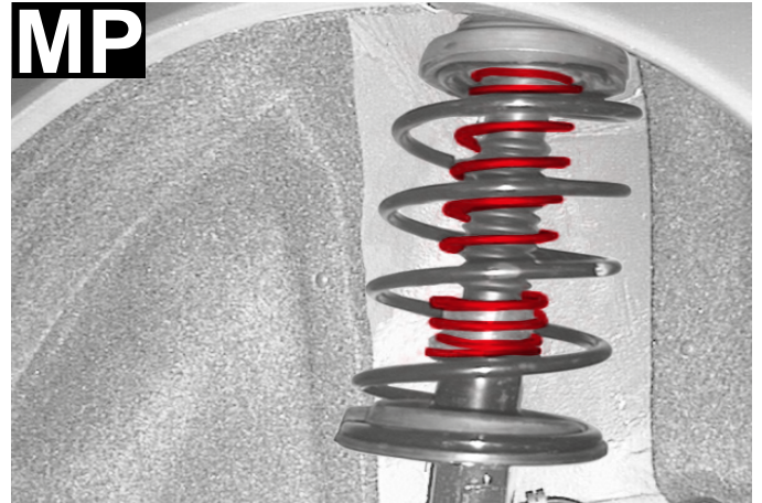
MP Sulla sospensione portante On the load suspension system Auf dem Federbein - Sur le support de suspension En la suspensión original - In het mc pherson systeem
