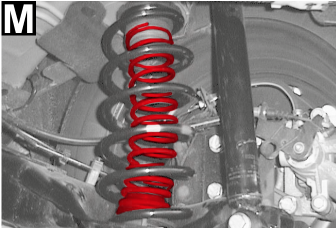
M Interna al mollone originale Inside the original suspension spring In der Originalfeder - A l'intérieur du ressort existant Al interno muelles originales - In de hoofveer
