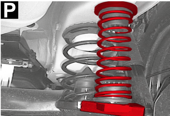
P Tra il ponte della ruota e la carrozzeria - Between the rear axle and chassis - Zwischen Achse und Karosserie - Entre le pont arrière et la carrosserie - Sobre el puente de la carroceria Tussen de achteras en chassis
